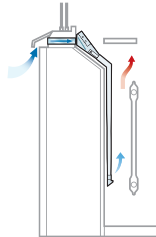
Installation med luftdon Flexi-SVK placerad över befintlig håltagning i fönsterkarmens underkant
