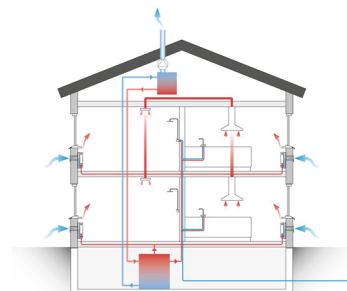
FX-VP system med Easy-Vent® FX bakom radiatorer.
