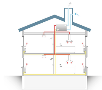
FTX-system med Easy-Vent® FTX bakom radiatorn med bjälklagsförlagda tilluftskanaler.
