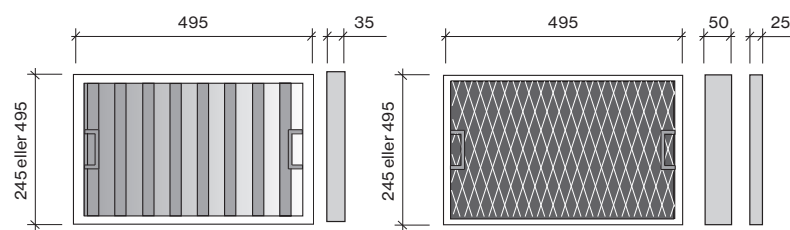
Flamskyddsfilter F finns i två storlekar, 500x250 och 500x500 mm. Filtret är 35 mm tjockt.
