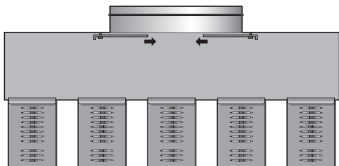
Figur 11 - Mätspjället är placerat i filterhuset strax under stosöppningen. Spjällbladen skjuts i sidled
